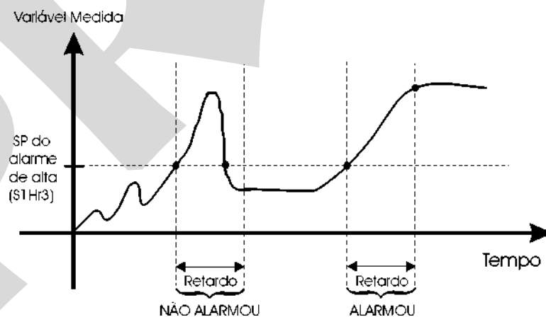
Fig.16 - Relé com Retardo
