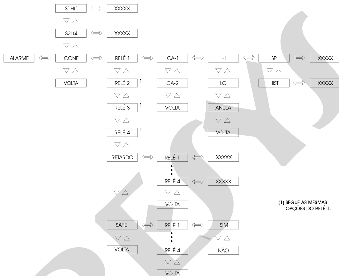
Fig. 17 - Opções do nível ALARME
