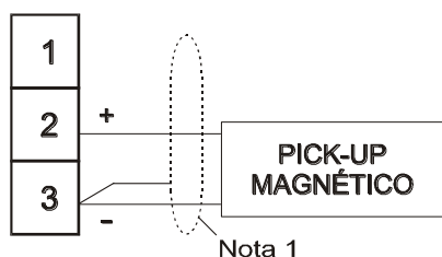
PICK-UP MAGNÉTICO
