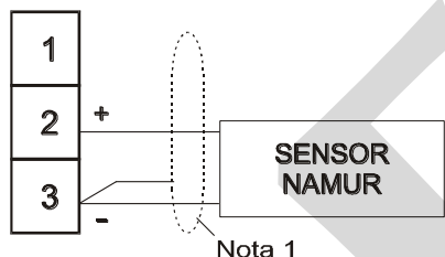
SENSOR NAMUR (pull-up interno de 866 \Omega ligado a +8V obtido ao colocar na Placa da CPU jumper JS1 para Entrada 1 ou JS2 para Entrada 2)
