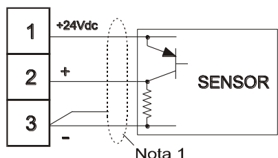
SENSOR COM SAÍDA A COLETOR ABERTO PNP (Sensores de proximidade indutivos, capacitivos, ópticos, etc.)
