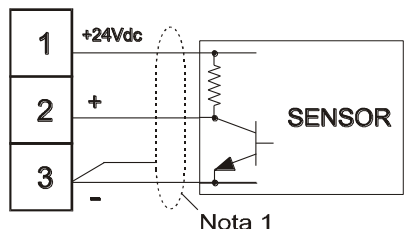
SENSOR COM SAÍDA A COLETOR ABERTO NPN (Sensores de proximidade indutivos, capacitivos, ópticos, etc.)
