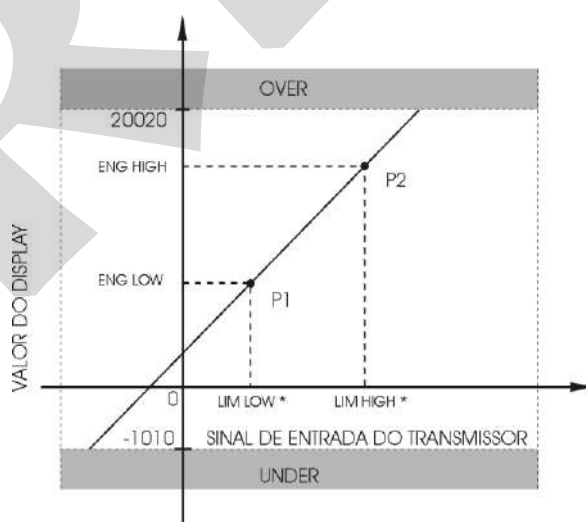
Fig. 13 - Configuração das entradas lineares
