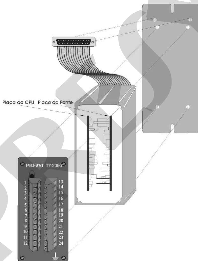
Fig. 19 - Esquema para desmontagem do instrumento
