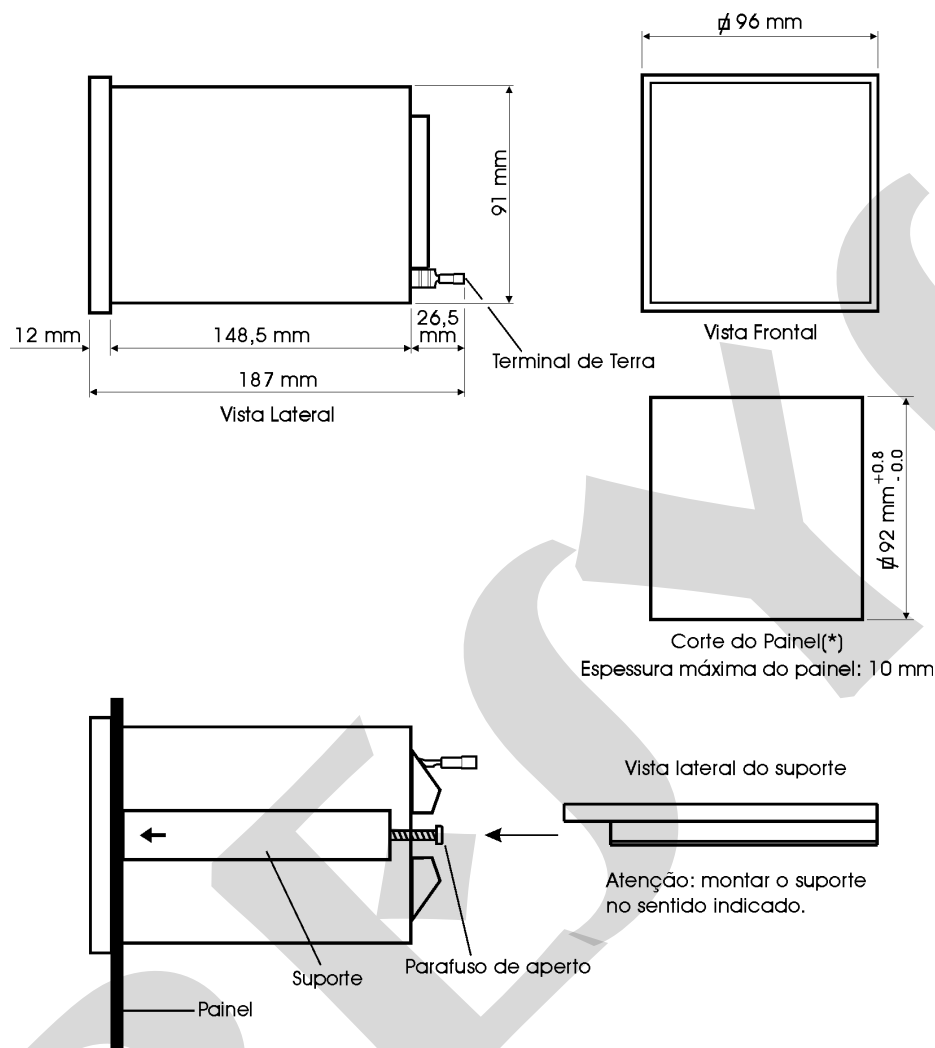
Fig. 4 - Desenho dimensional, corte e vista lateral da montagem no painel do Indicador SCY - 2011
