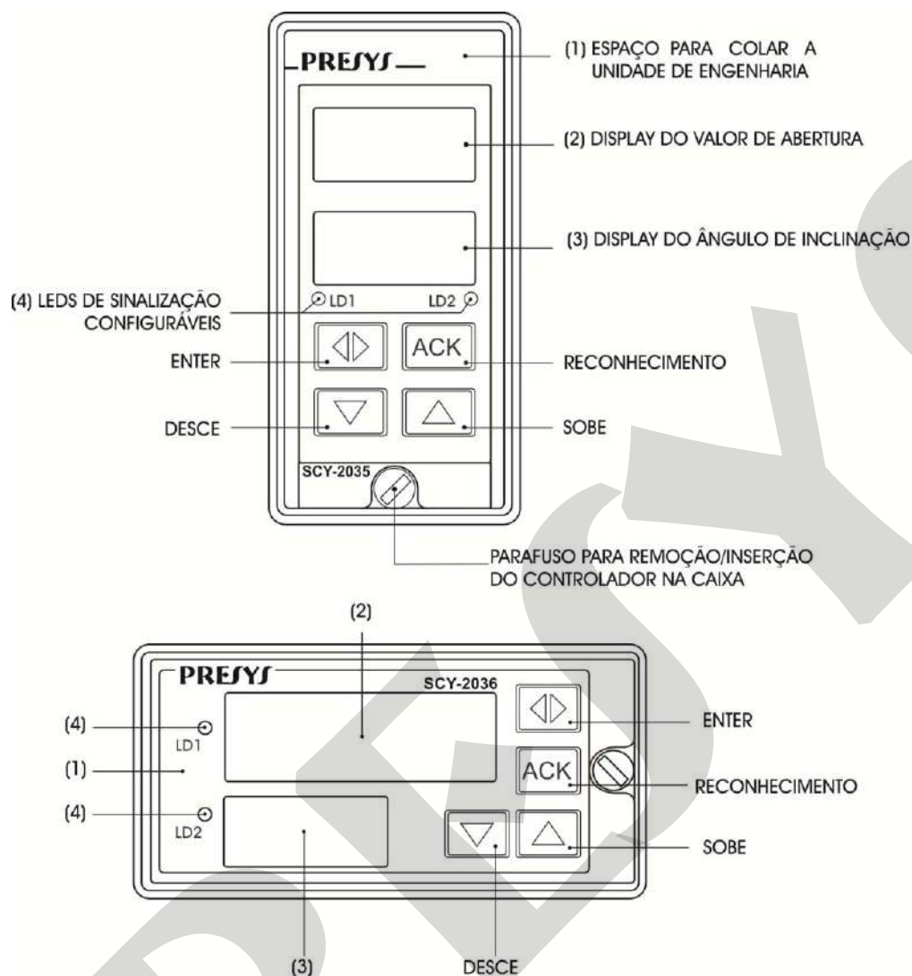
Fig. 2 - Painel frontal dos Indicadores SCY-2035 e 2036
