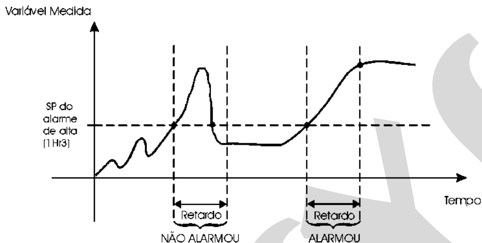
Fig. 16 - Relé com Retardo
