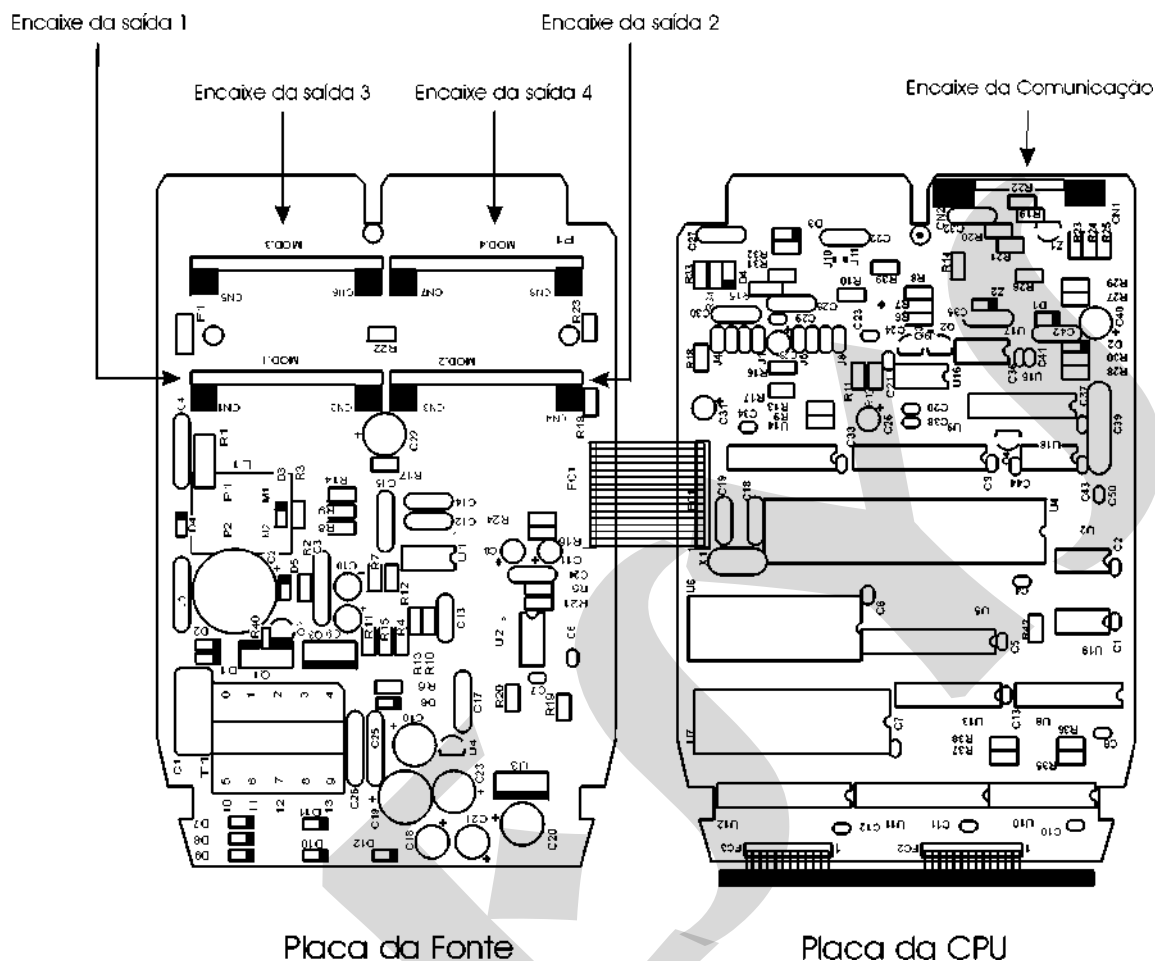
Fig. 21 - Encaixes dos módulos
