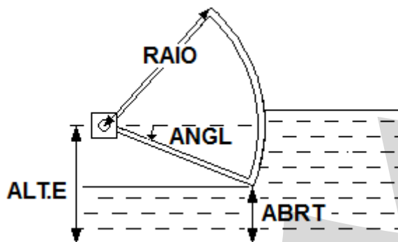
Fig. 12 - Relação dos parâmetros ALT.E e RAIO do nível ABERTURA e do ângulo de inclinação ANGL com a abertura ABRT da comporta.
