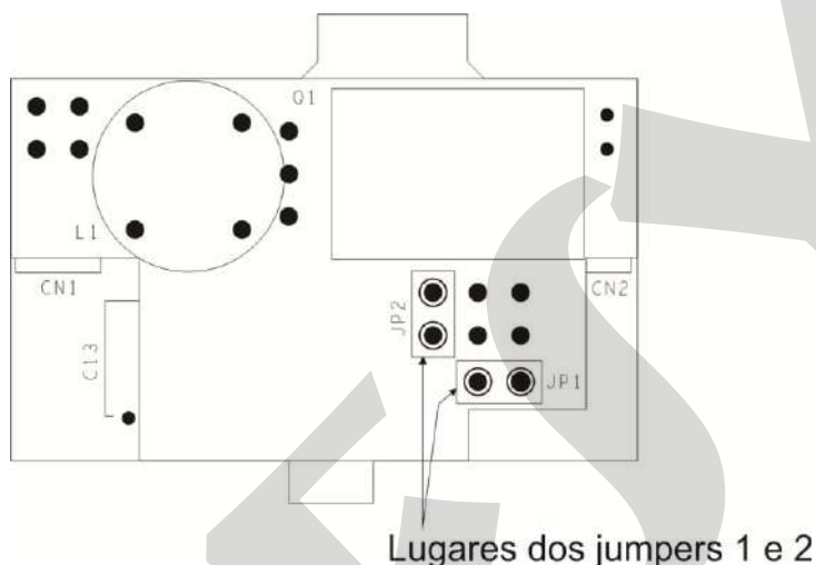
Fig. 23 - Localização dos lugares dos jumpers na placa de saída analógica
