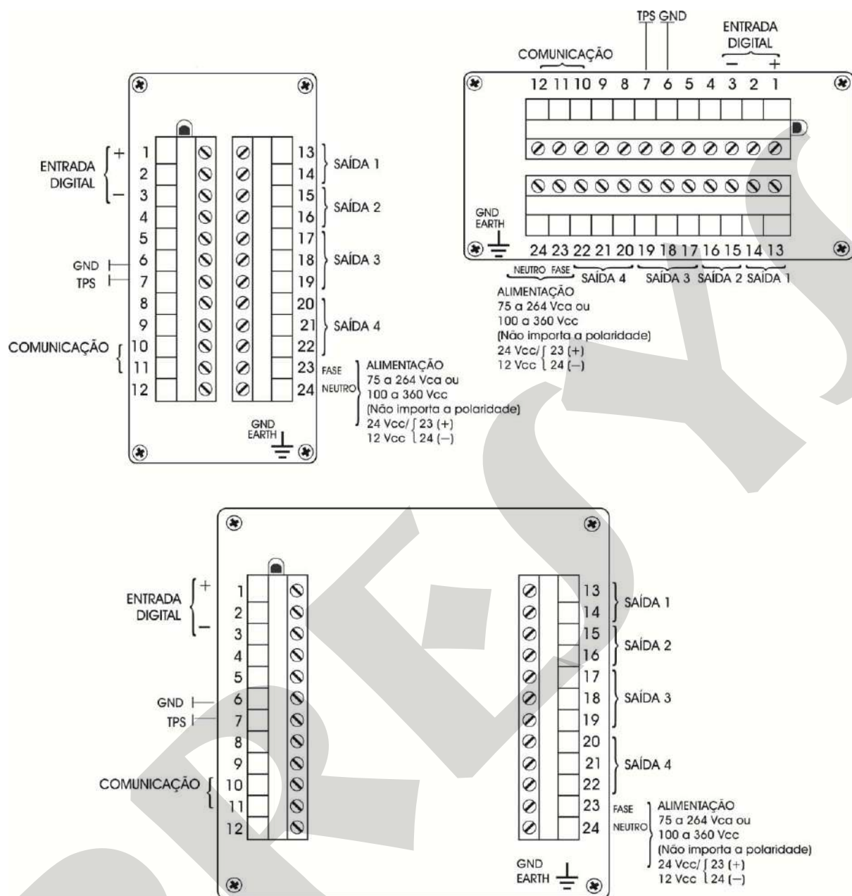
Fig. 5 - Borneira dos Indicadores
