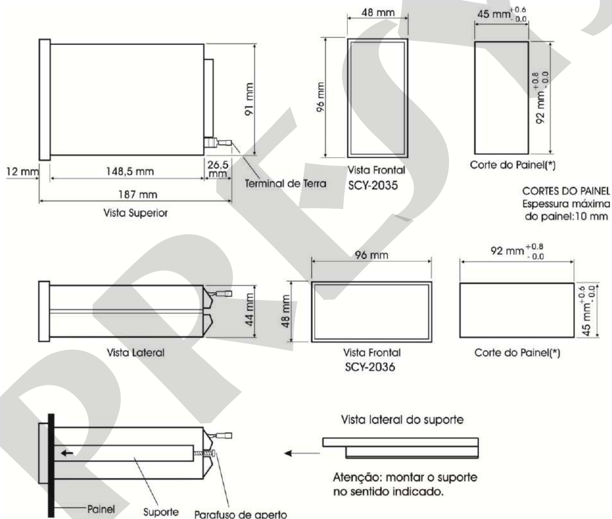
Fig. 3 - Desenho dimensional, corte e vista lateral da montagem no painel dos Indicadores SCY - 2035 e 2036
