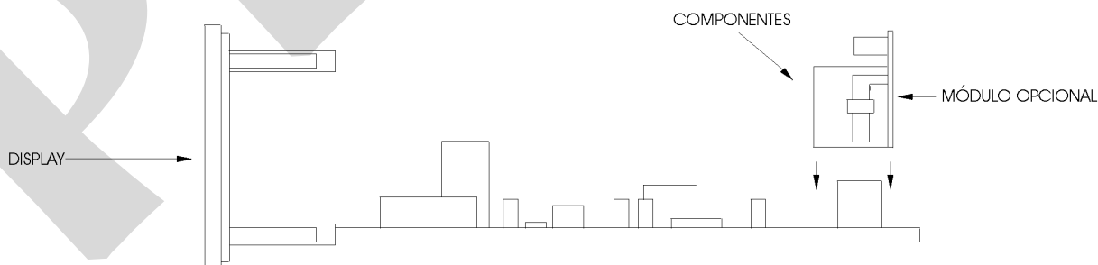
Fig. 22 - Instalação dos módulos opcionais de saída
