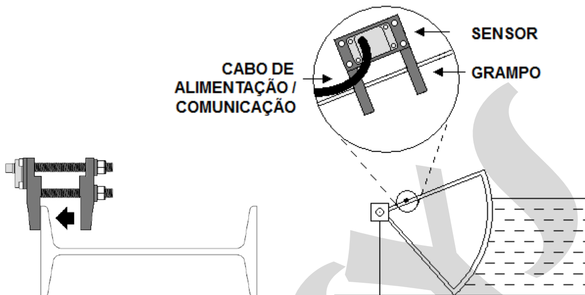
Fig. 6 – Fixação do grampo à viga e posicionamento do suporte no braço da comporta
