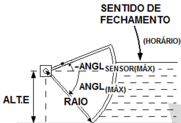
Fig. 14 – Relação da geometria da comporta fechada com os parâmetros ALT.E e RAI0 e dos valores máximos dos ângulos de inclinação ANGL e de leitura do sensor ANGL SENSOR .
