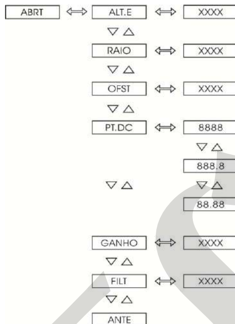
Fig. 11 - Opções do nível ENTRADAS
