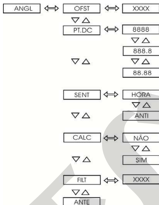
Fig. 13 - Opções do nível ÂNGULO
