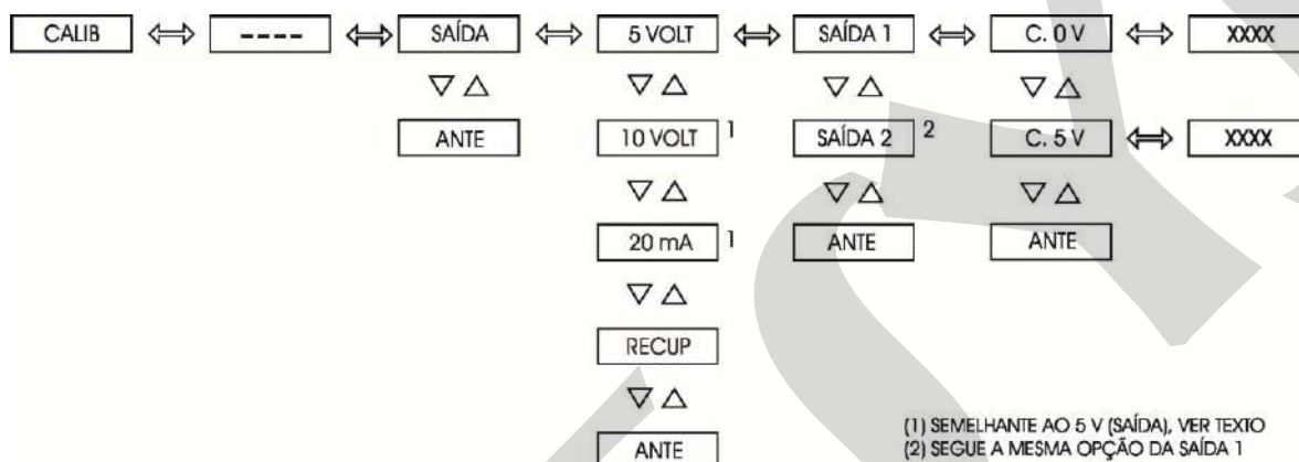
Fig. 24 - Opções do nível CALIBRAÇÃO
