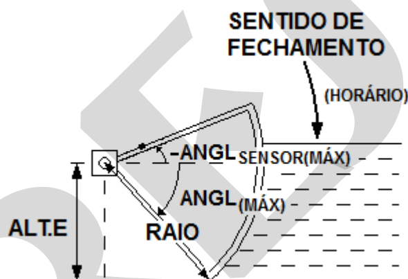
Fig. 15 - Relação da geometria da comporta fechada com os parâmetros ALT.E e RAI0 e dos valores máximos dos ângulos de inclinação ANGL e de leitura do sensor ANGL_{SENSOR} .
