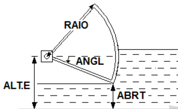
Fig. 13 - Relação dos parâmetros ALT.E e RAIO do nível ABERTURA e do ângulo de inclinação ANGL com a abertura ABRT da comporta.
