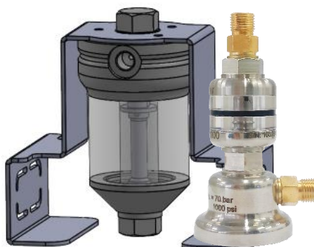
Fig. 113 - Separadores de Impurezas SI-600, SI-1000 e SI-3000
