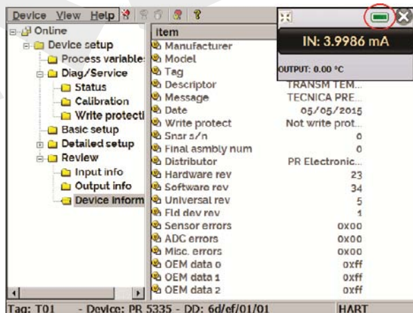
Fig. 70 - Valores de Entrada e Saída do Calibrador / Controlador
