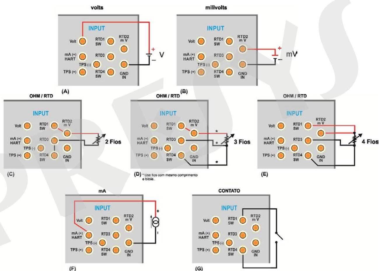
Fig. 41 - Conexões da Entrada Auxiliar
