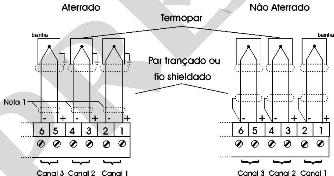
Fig. 4 - Conexão de termopares
