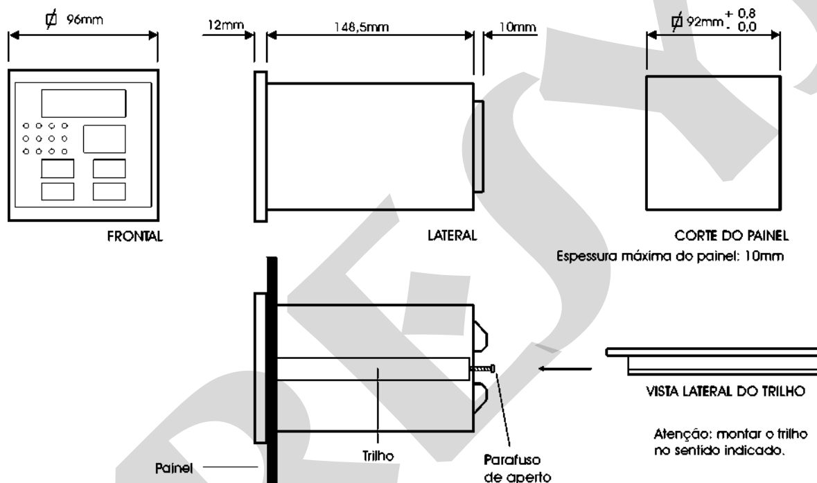
Fig. 2 - Desenho dimensional, corte e vista lateral da montagem no painel
