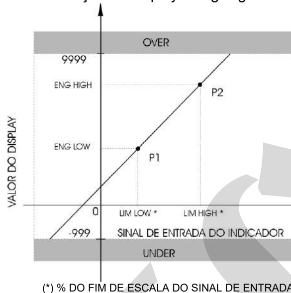
Fig.14 - Configuração das entradas lineares
