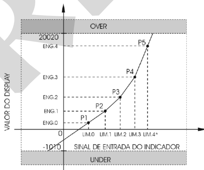
Fig. 12 - Configuração da entrada linear
