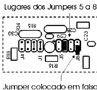
Fig. 21 – Jumper colocado em falso para a entrada de 0 a 10 V do canal 1
