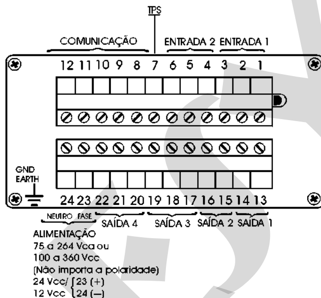
Fig. 3 - Borneira do Indicador
