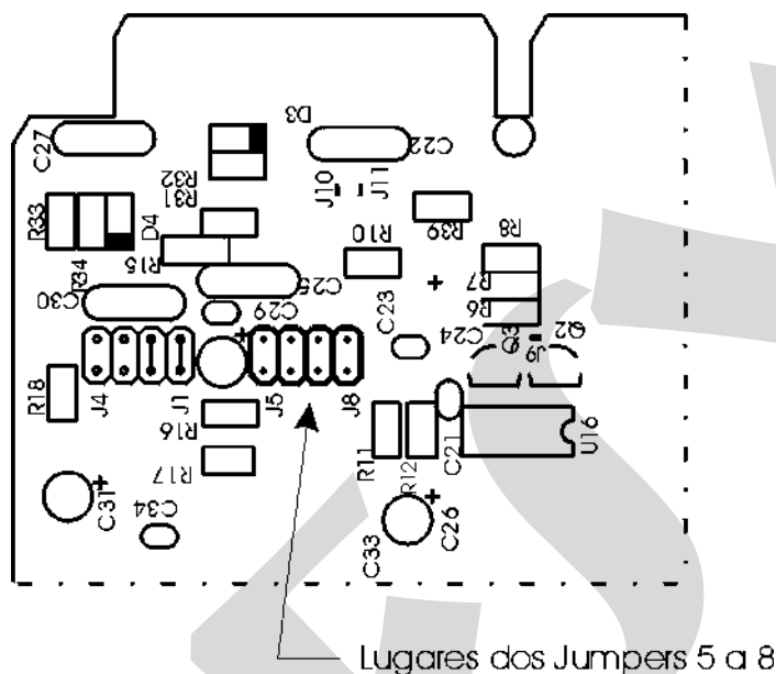
Fig. 20 - Localização dos lugares dos jumpers na Placa da CPU
