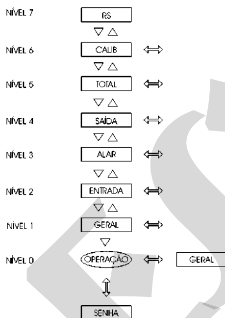
Fig. 9 - Diagrama dos níveis dos parâmetros
