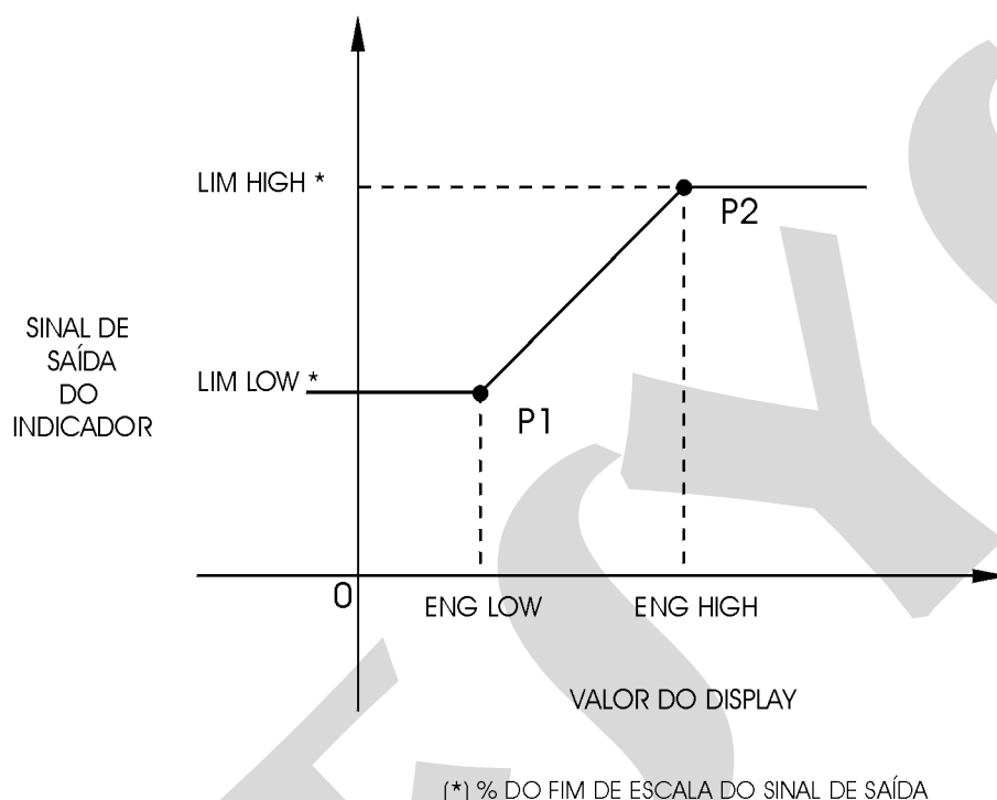
Fig. 16 - Configuração das saídas analógicas
