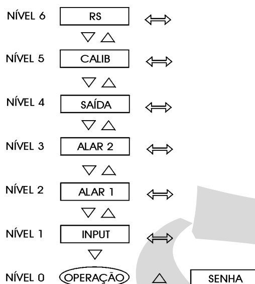
Fig. 11 - Diagrama dos níveis dos parâmetros
