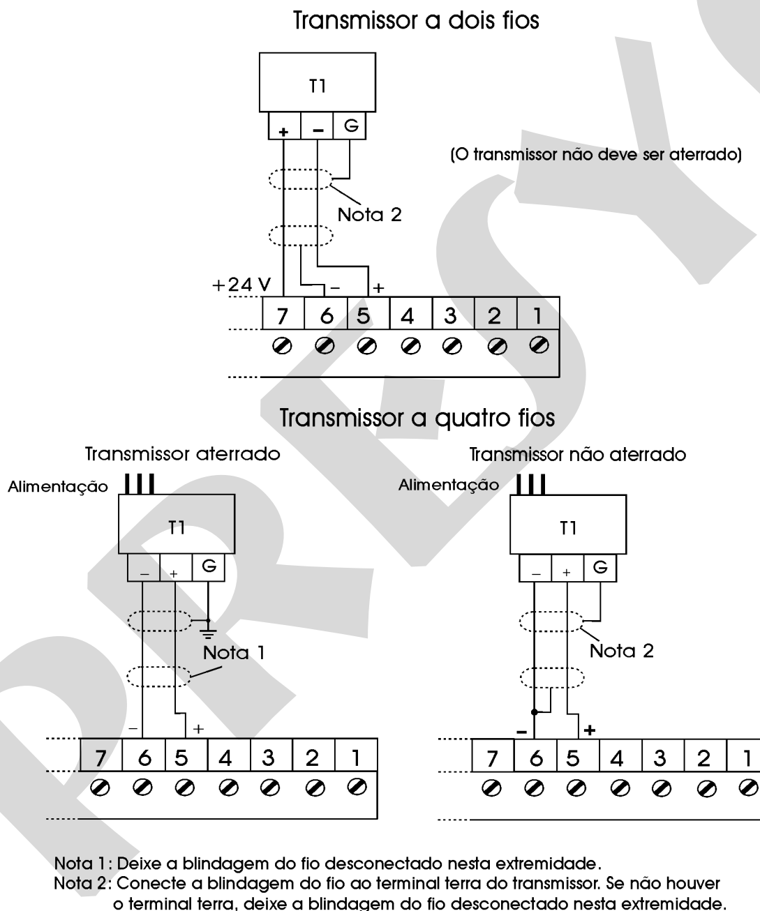
Fig. 6 - Conexão da fonte de corrente
