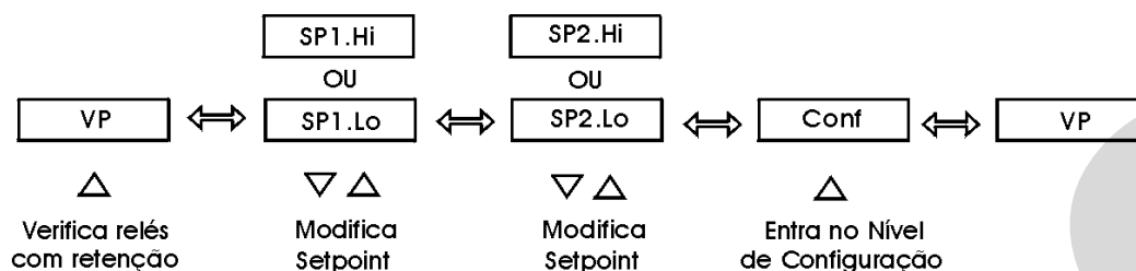
Fig. 9 - Informações do nível de operação.
