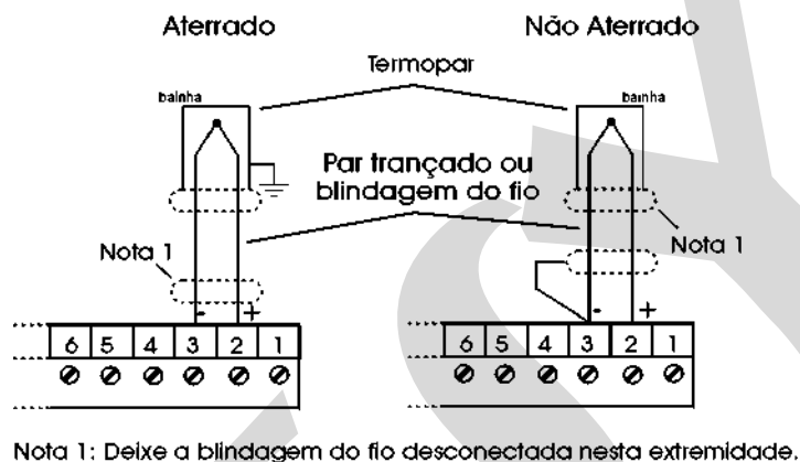
Fig. 4 - Conexão de termopar
