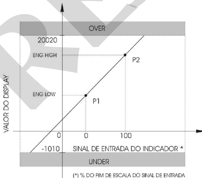
Fig. 13 - Configuração da entrada linear
