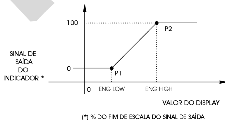
Fig. 18 - Configuração da saída analógica
