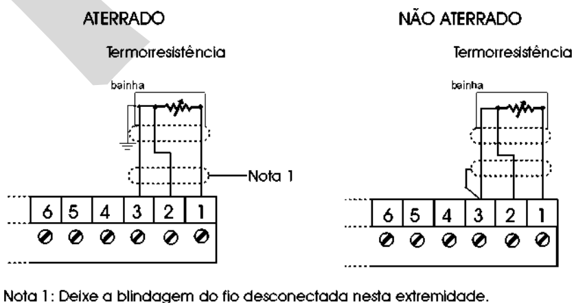
Fig. 5 - Conexão de termorresistência
