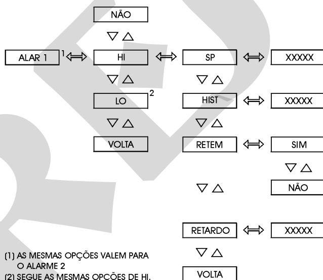
Fig. 15 - Opções dos níveis ALARME 1 e ALARME 2
