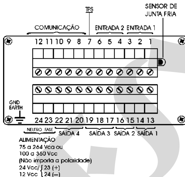
Fig. 3 - Borneira do Indicador
