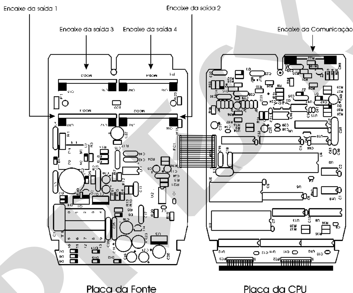
Fig. 23 - Encaixes dos módulos opcionais
