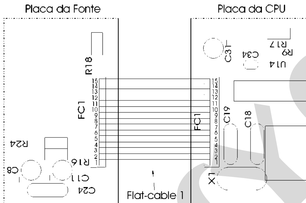
Fig. 27 - Pontos de teste de tensão do Indicador
