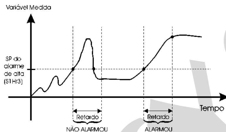
Fig. 15 - Relé com Retardo
