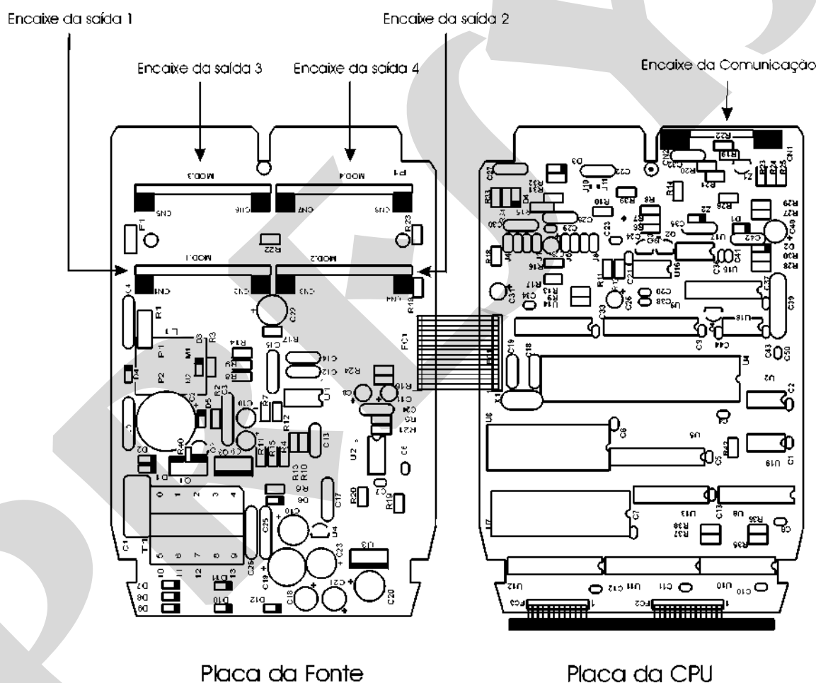
Fig. 25 - Encaixes dos módulos opcionais
