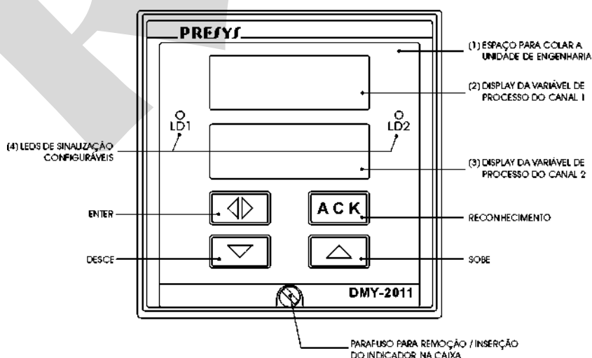
Fig. 1 - Painel frontal do Indicador duplo DMY-2011
