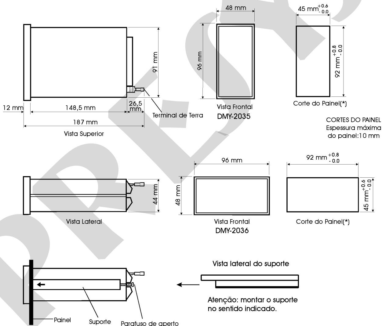
Fig. 3 - Desenho dimensional, corte e vista lateral da montagem no painel dos Indicadores DMY - 2035 e 2036
