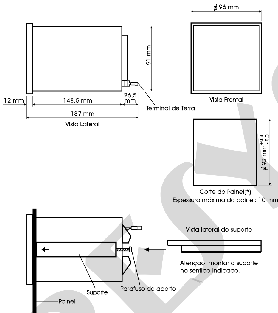
Fig. 4 - Desenho dimensional, corte e vista lateral da montagem no painel do Indicador DMY - 2011
