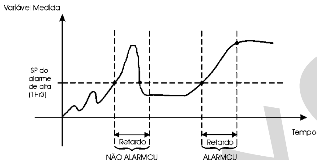
Fig. 17 - Relé com Retardo
