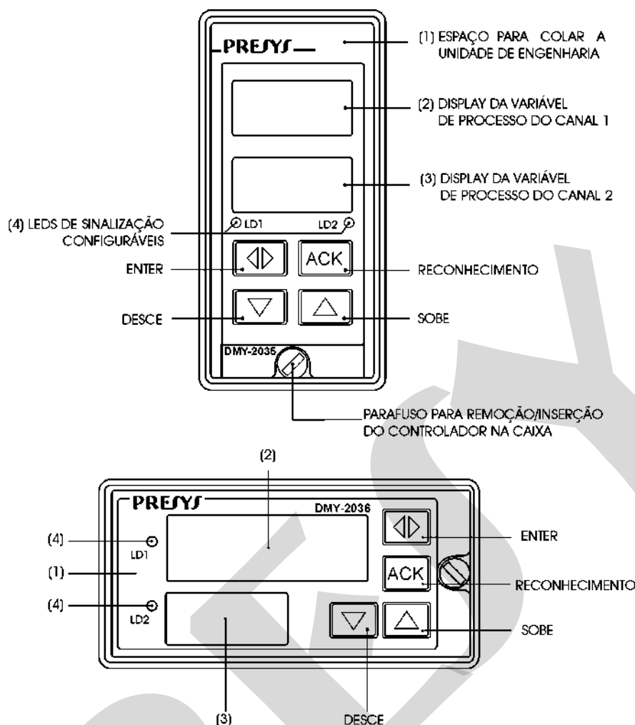
Fig. 2 - Painel frontal dos Indicadores duplos DMY-2035 e 2036
