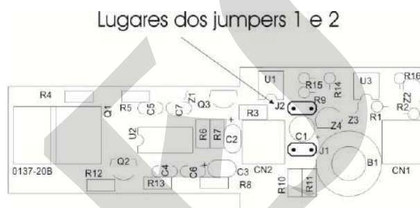
Fig. 24 - Localização dos jumpers na placa de saída analógica
