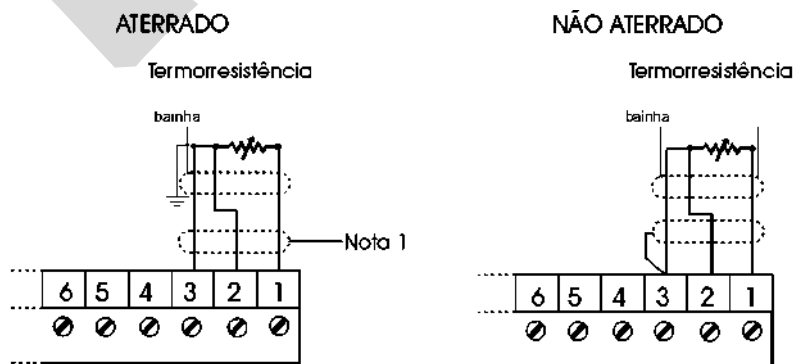
Fig. 5 - Conexão de termorresistência
