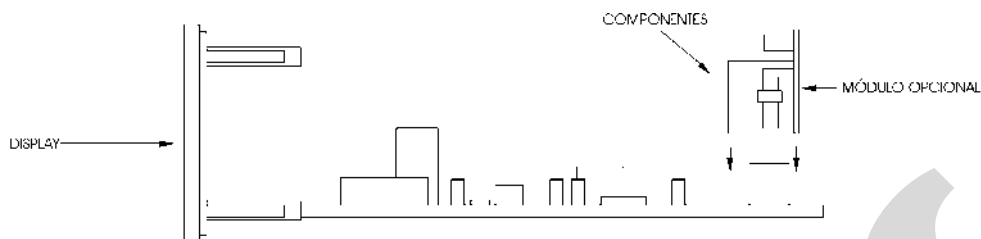
Fig. 23 - Instalação dos módulos opcionais
