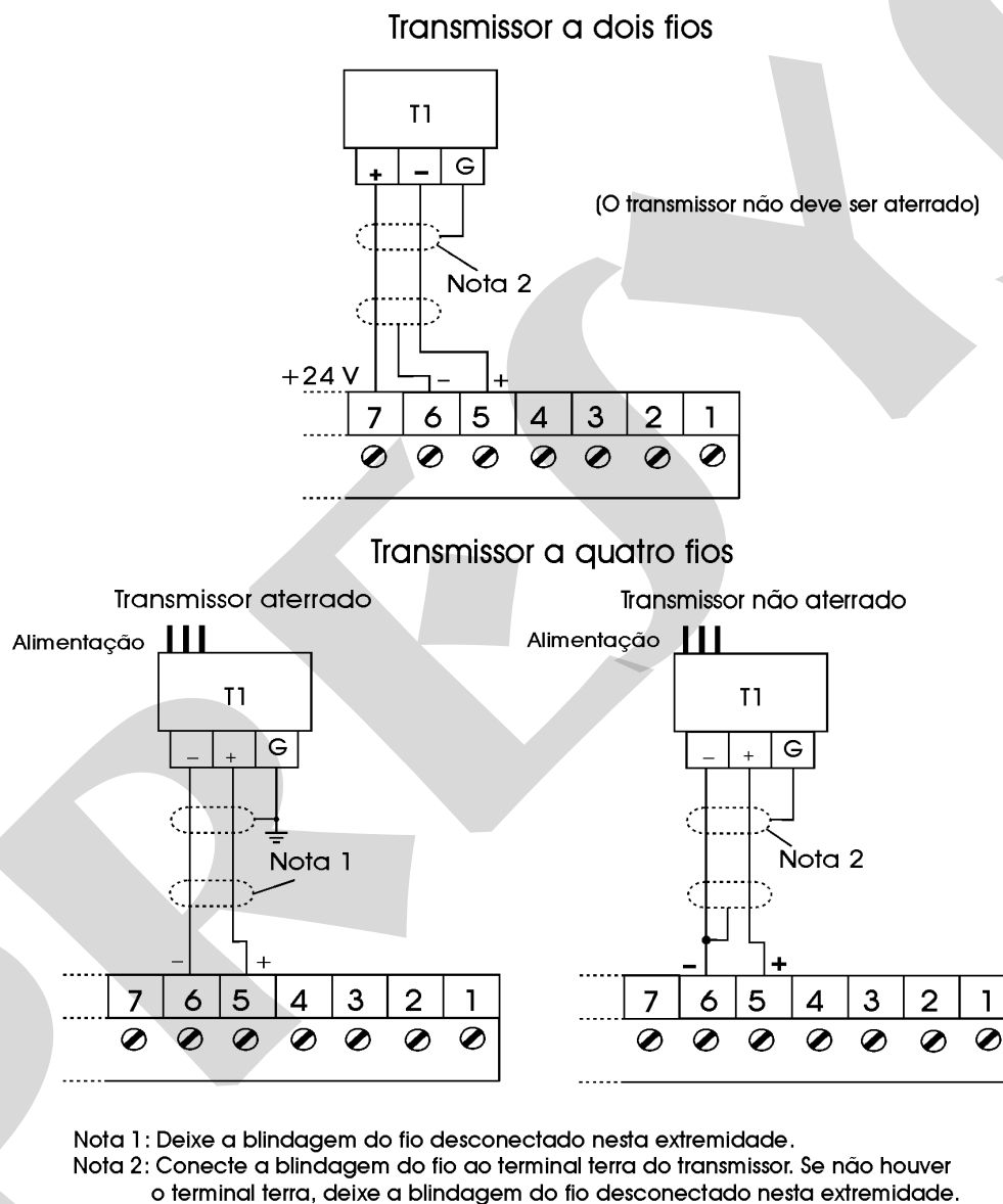
Fig. 6 - Conexão da fonte de corrente
