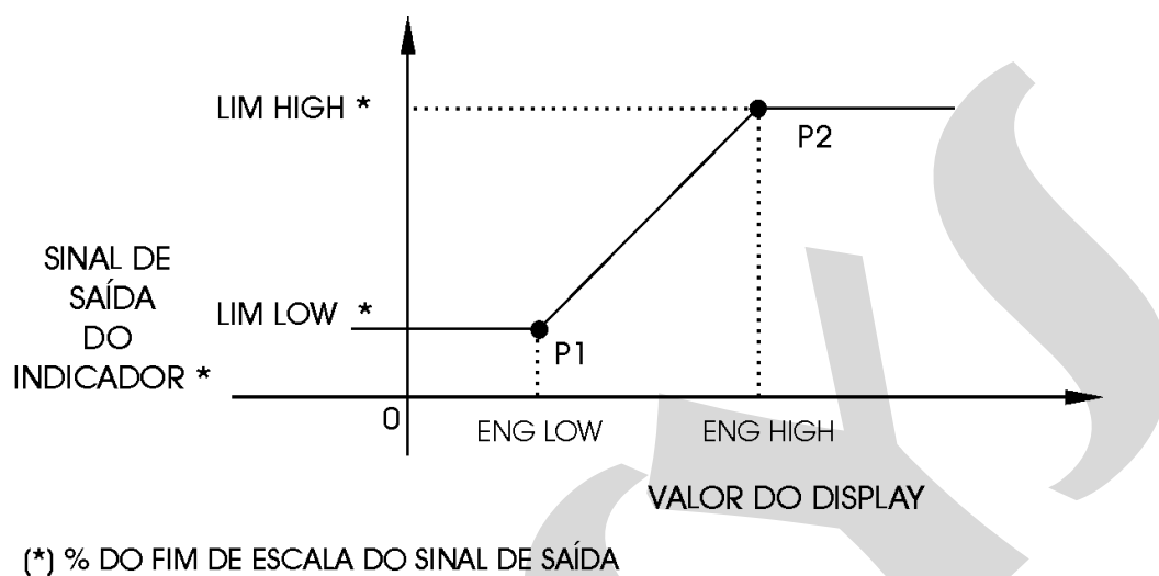
Fig. 18 - Configuração das saídas analógicas
