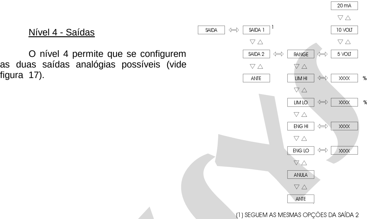
Fig. 17 - Opções do nível SAÍDAS
