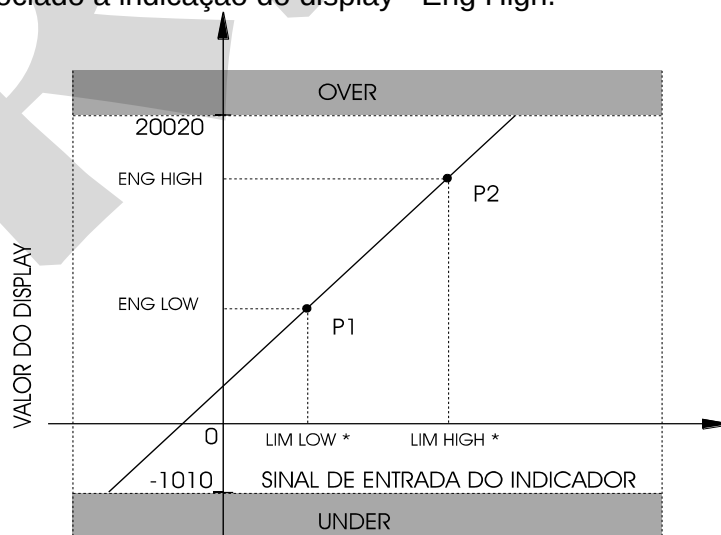
Fig. 13 - Configuração das entradas lineares Fig. 14 - Configuração das entradas lineares
