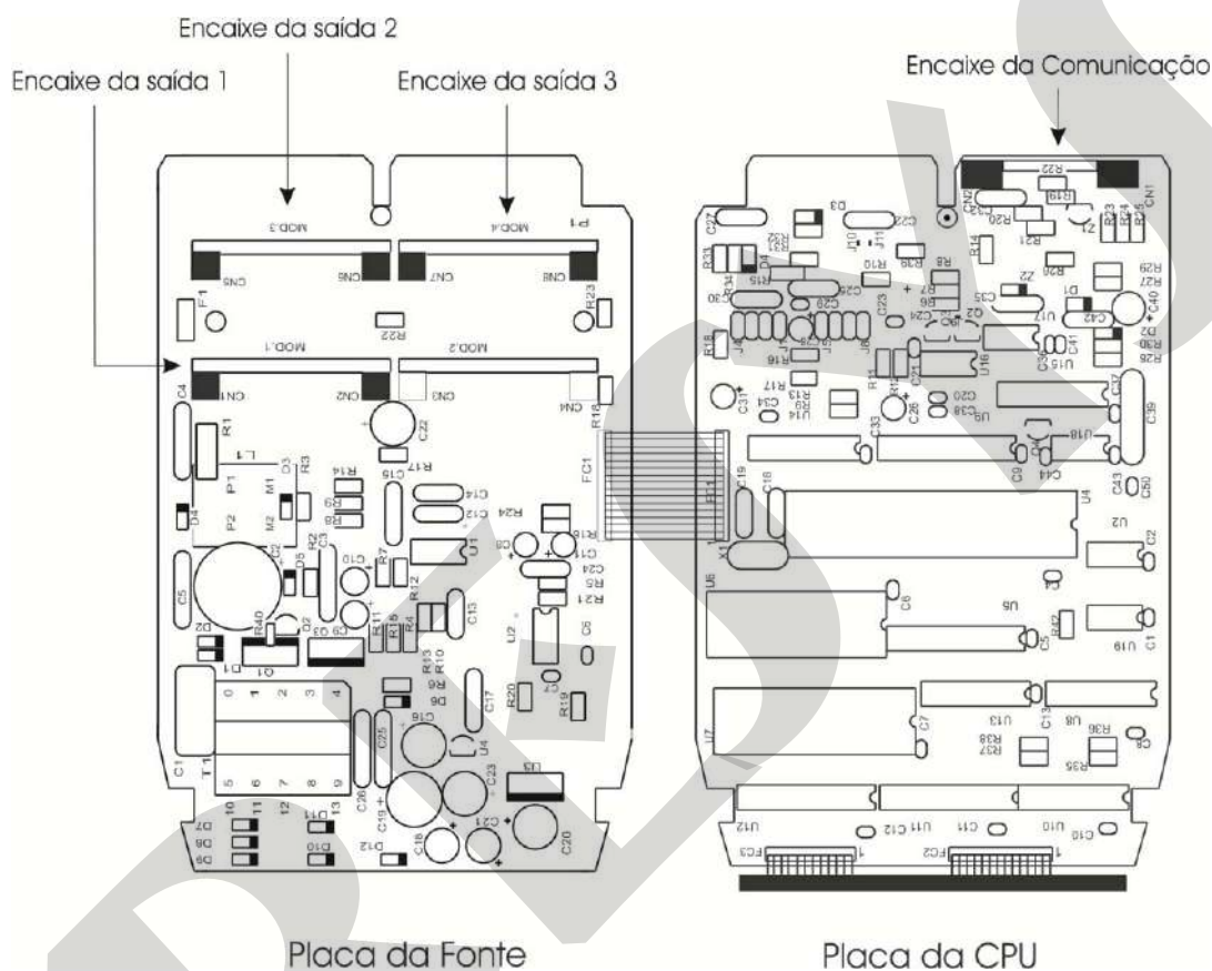
Fig. 19 - Encaixes dos módulos opcionais
