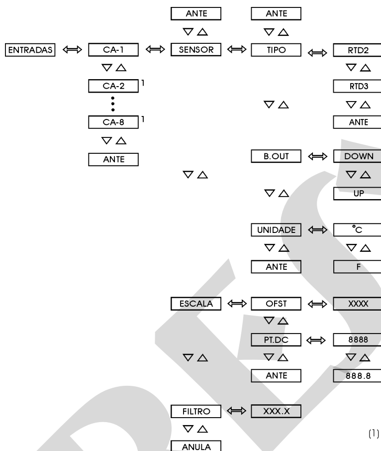
Fig. 10 - Opções do nível ENTRADAS
