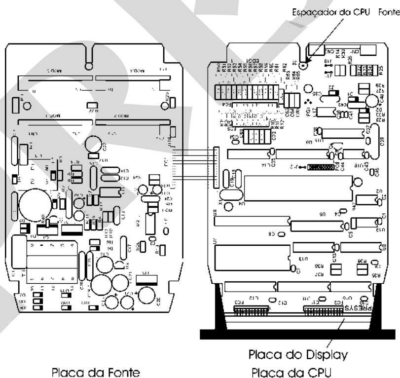
Fig.13 - Hardware do Indicador
