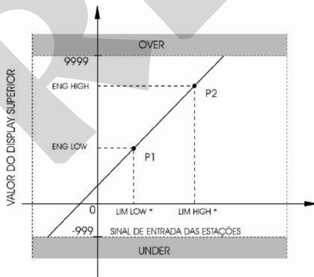
Fig. 12 - Configuração das entradas lineares
