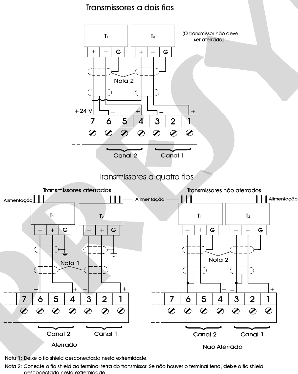
Fig. 4 - Conexão da fonte de corrente
