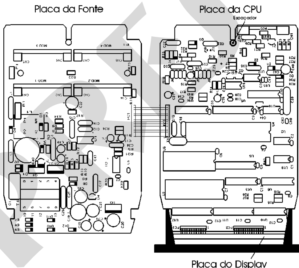
Fig. 33 - Hardware dos controladores
