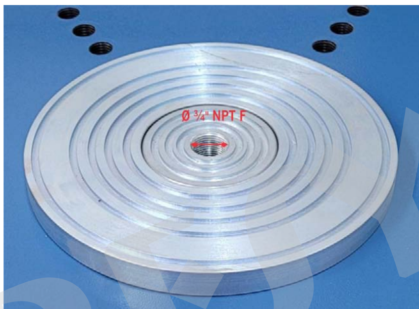
Fig. 18 - Flange Central com Rosca Fêmea NPT de \frac{3}{4} "
