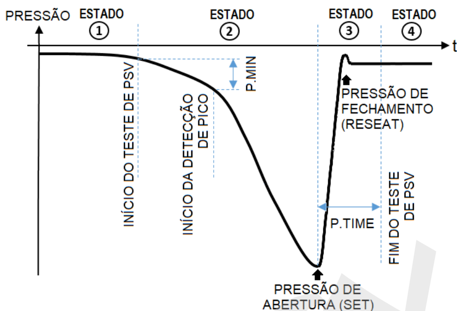
Fig. 33 - Ciclo de teste de válvulas PSV (continuação)
