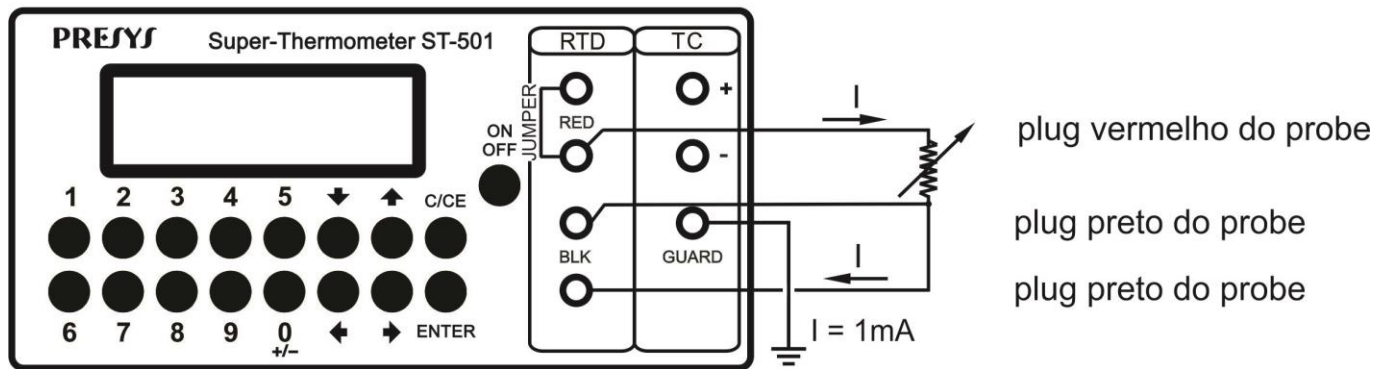
Fig. 3 - Conexões de entrada ou medição (3 fios)
