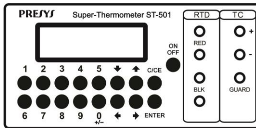
Fig. 5 - Calibração de Entradas
