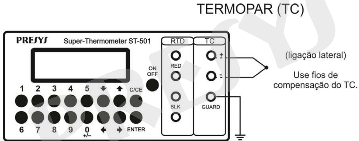
Fig. 4 – Conexões de entrada ou medição (Thermopar)
