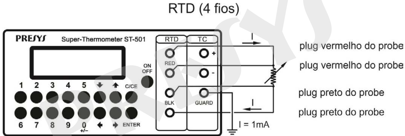
Fig. 2 – Ligações de Entrada ou Medição (4 fios)
