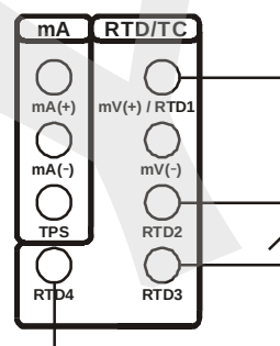
Ohm / RTD (4-fios)
