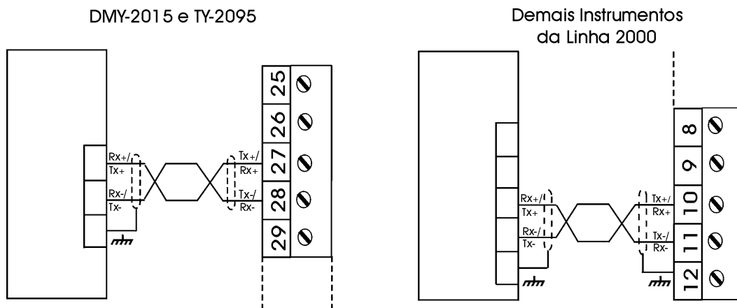
Fig. 4 - Ligação Elétrica para RS-485
