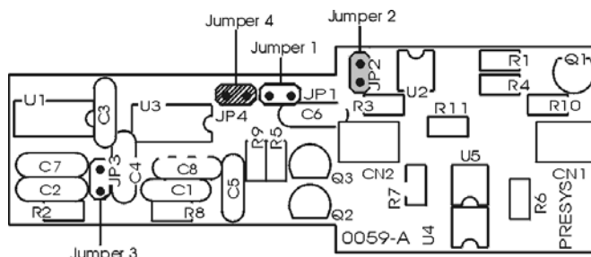
Fig. 5 - Módulo Opcional para RS-422 ou RS-485
