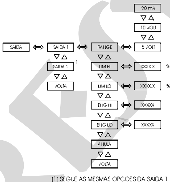
Fig. 16 - Opções do nível SAÍDAS
