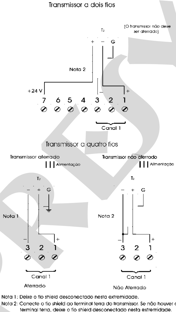
Fig. 4 - Conexão da fonte de corrente
