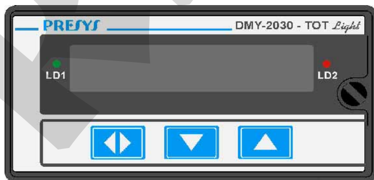
Fig. 1 - Painel frontal do Indicador Integrador e Totalizador DMY-2030-TOT Light
