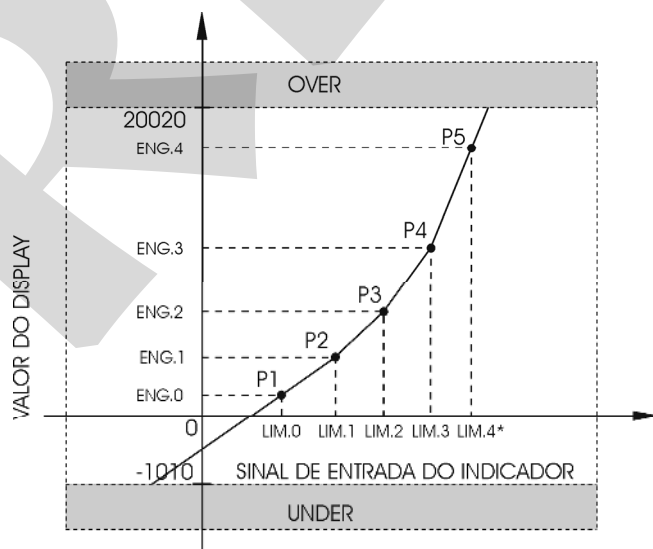
Fig. 12 - Configuração da entrada linear
