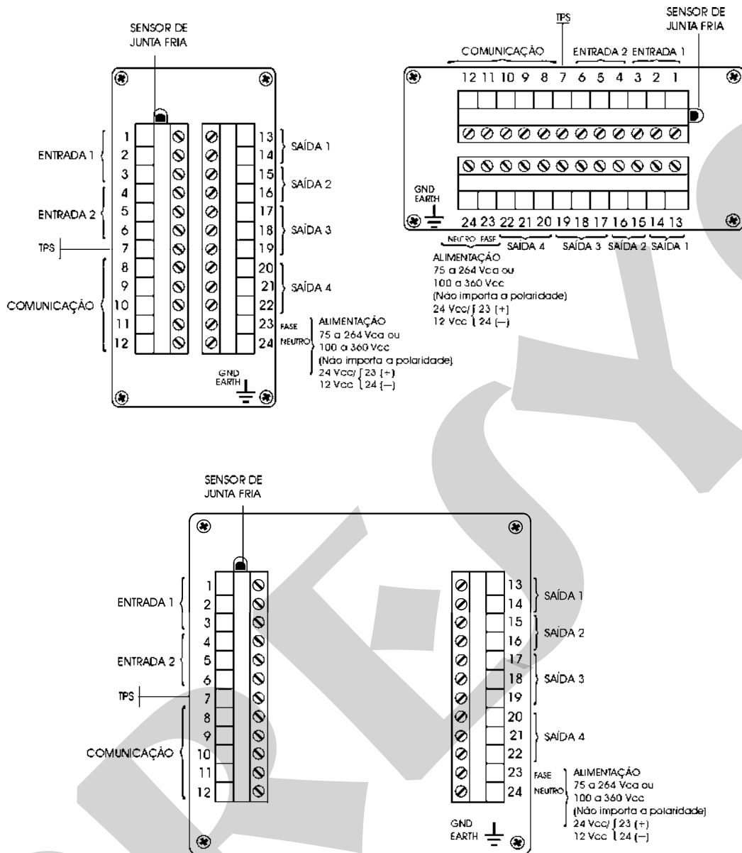
Fig. 5 - Borneira dos Indicadores
