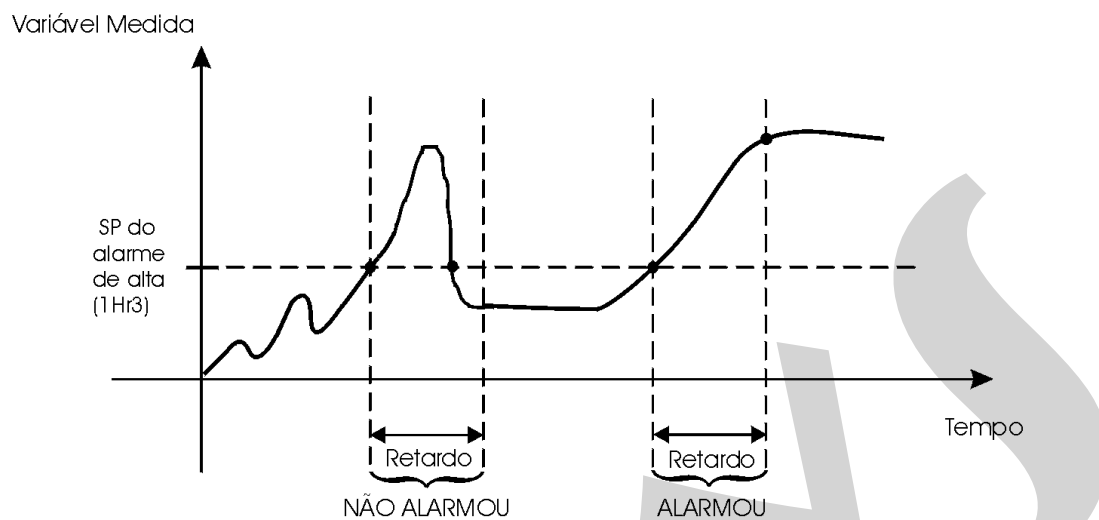
Fig. 17 - Relé com Retardo
