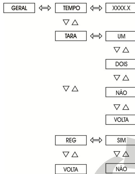
Fig. 16 - Opções do nível GERAL
