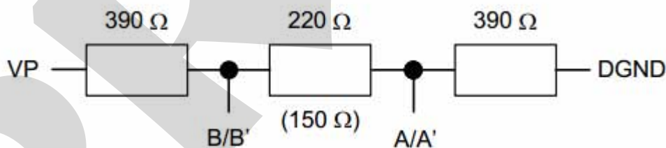
Fig.20 – Resistores de terminação
